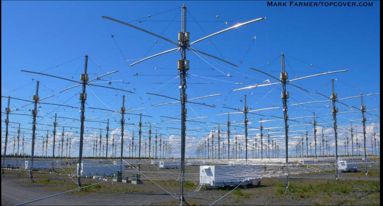
Typische HAARP KW-Antennenfelder
